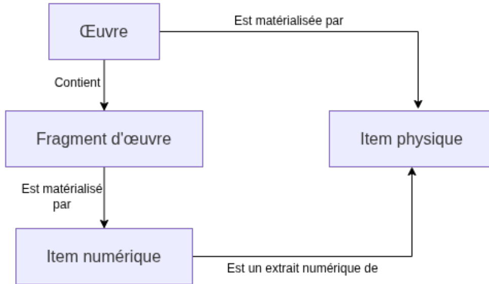
FIG. 3 : Intégration du Fragment au modèle de données
